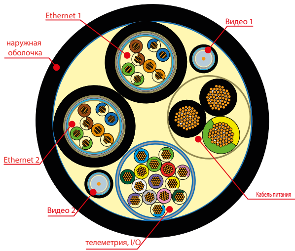
СЕЧЕНИЕ КАБЕЛЯ МРХСАВL
