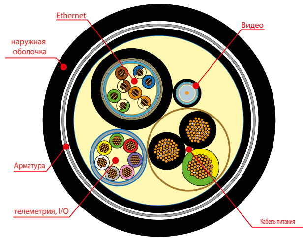
СЕЧЕНИЕ КАБЕЛЯ МРХСАВLARM
